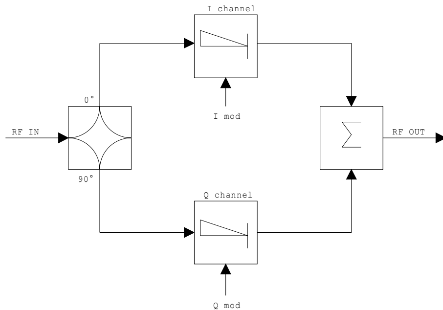
Fig. 4.27 I/Q modulation
